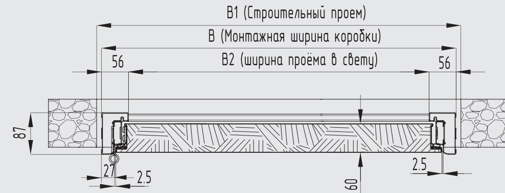
ДВЕРНАЯ КОРОБКА ДЛЯ ВРЕЗНОГО МОНТАЖА
