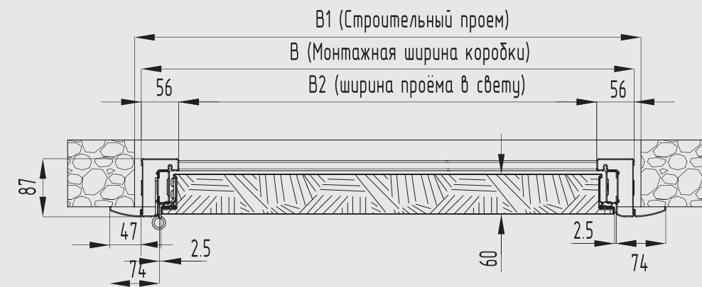
ДВЕРНАЯ КОРОБКА ДЛЯ НАКЛАДНОГО МОНТАЖА
